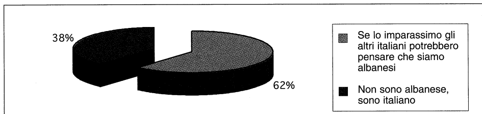
Figura 7. Inutilità dell’apprendimento.
